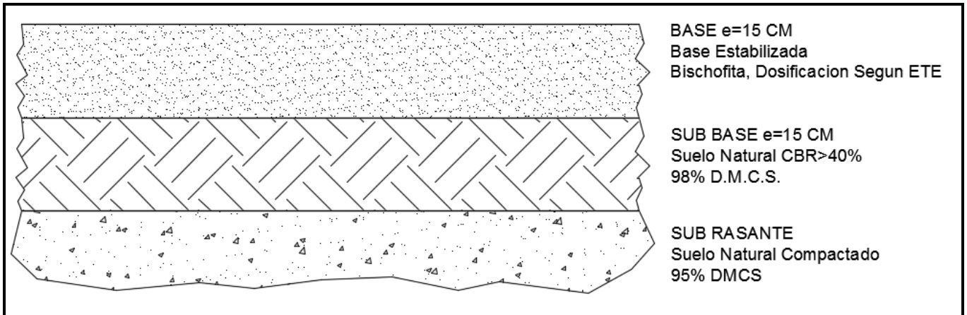
Imagen N°1.- Disposición de la Carpeta de Pavimento de Bischofita
